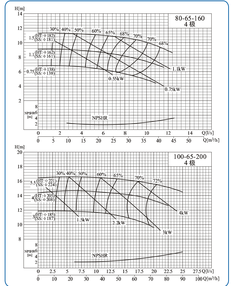
80-65-160/100-65-200
