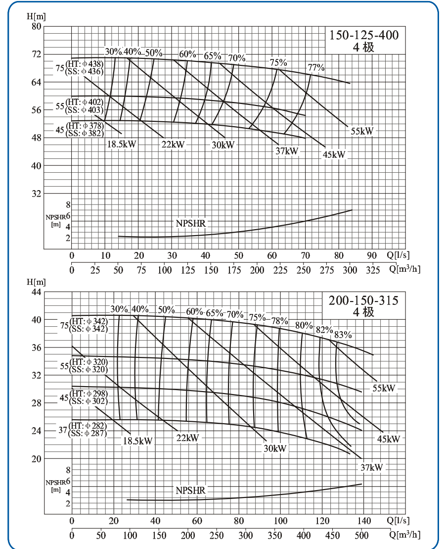
150-125-400/200-150-315
