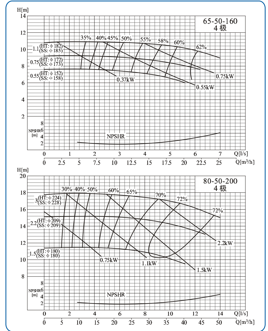
65-50-160/80-50-200
