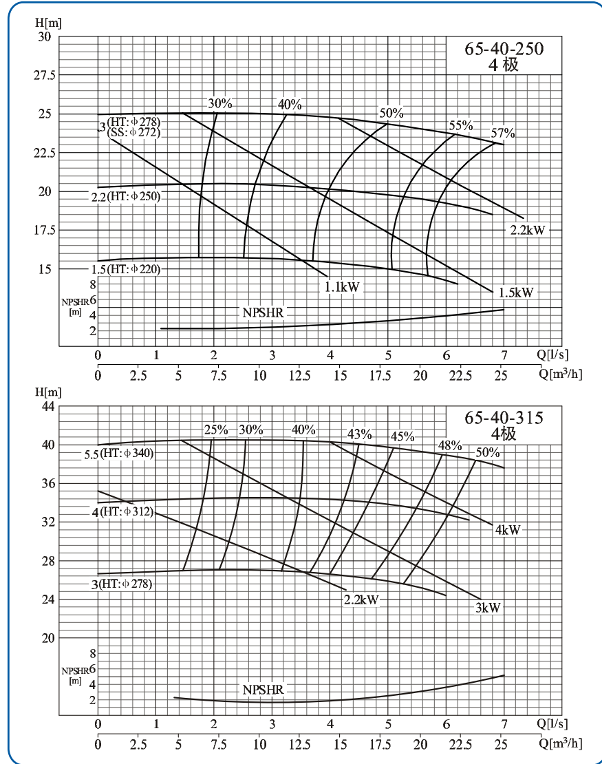
65-40-250/65-40-315
