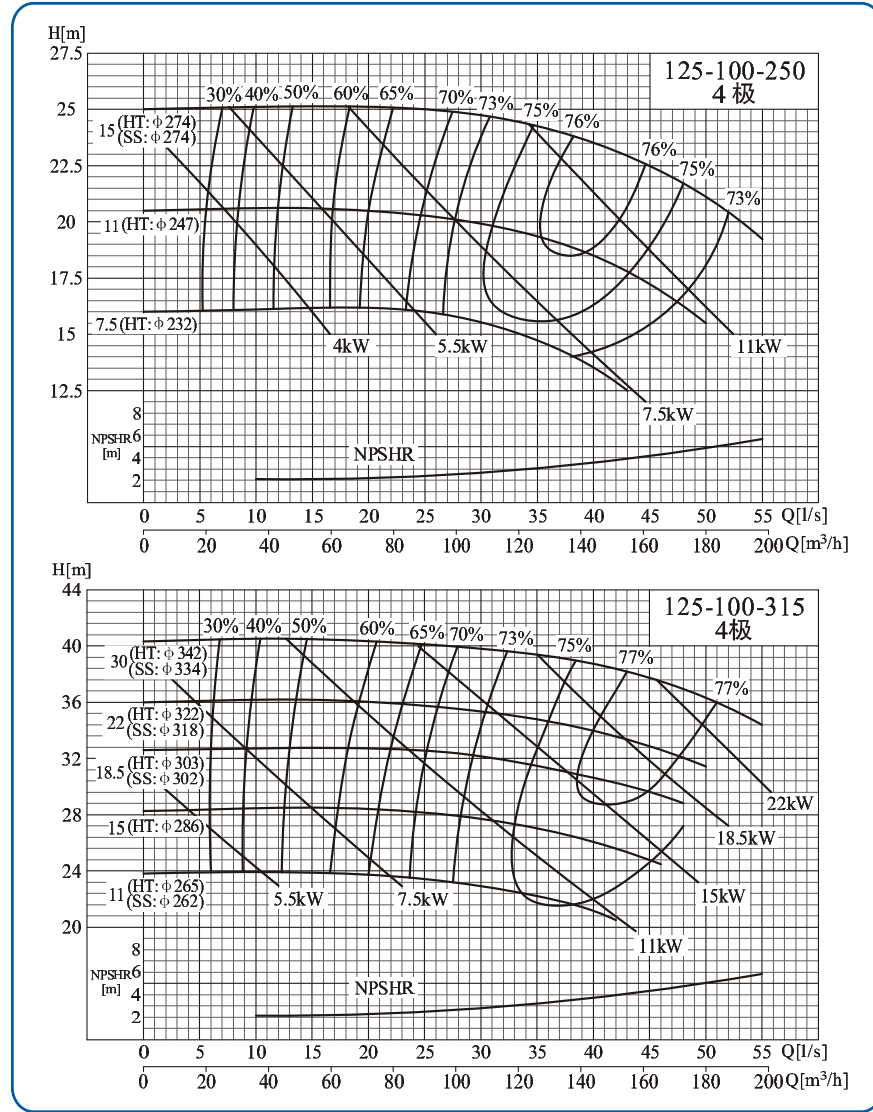
125-100-250/125-100-315
