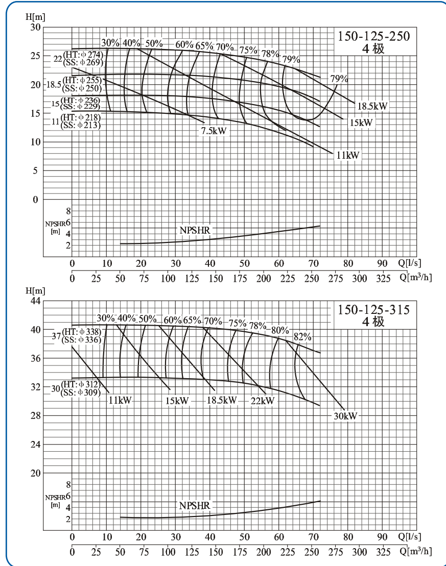
150-125-250/150-125-315
