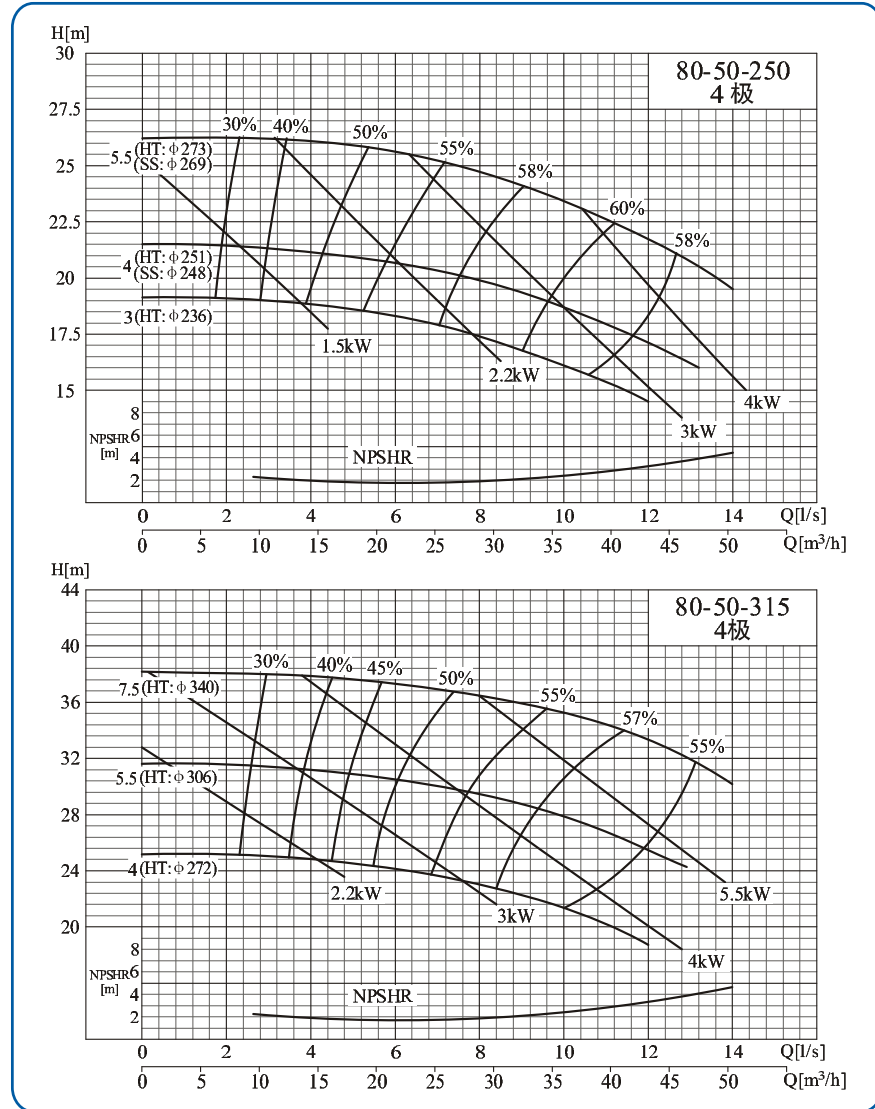
80-50-250/80-50-315
