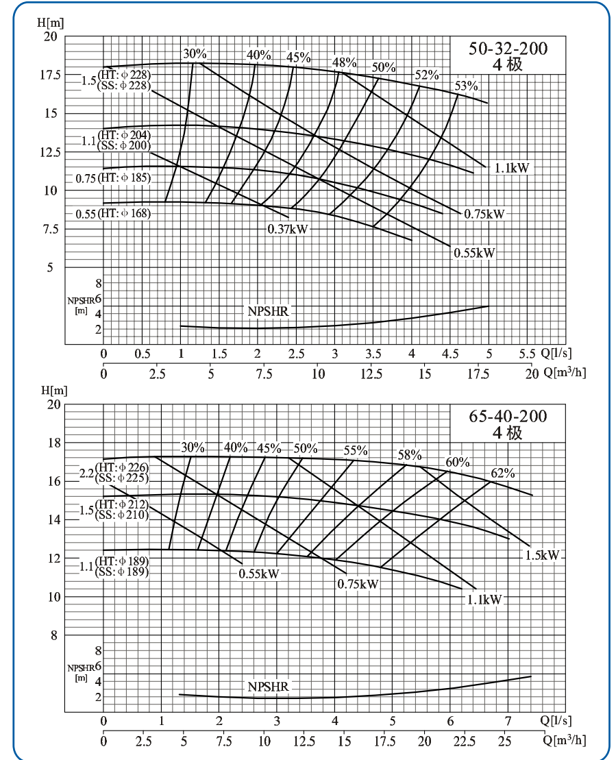
50-32-200/65-40-200
